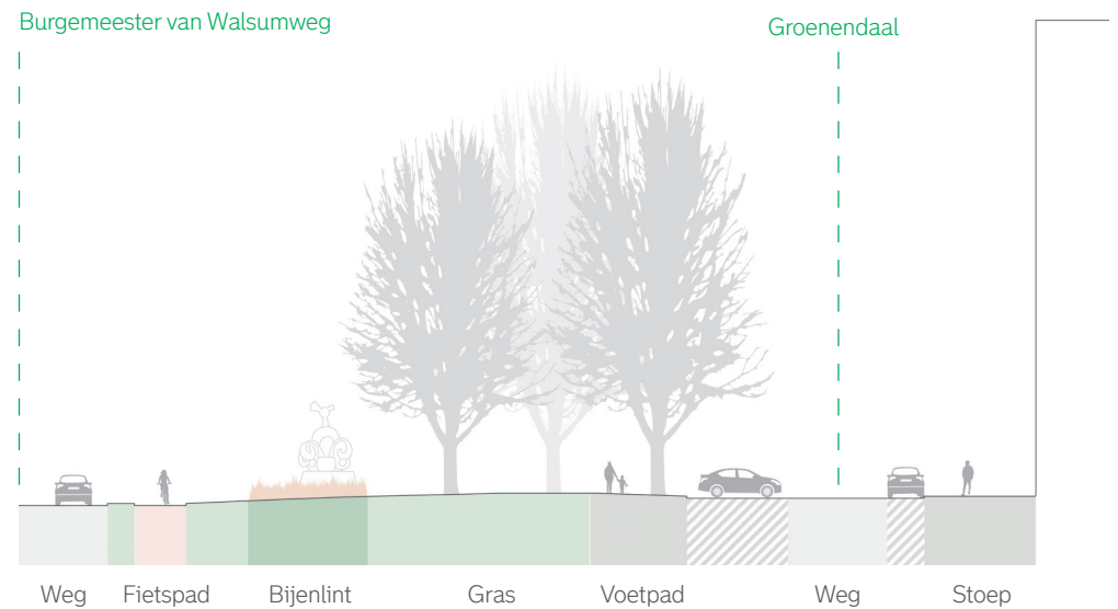
Een doorsnede vanaf de Burgemeester van Walsumweg tot aan de Groenendaal (Doorsnede 0b)
