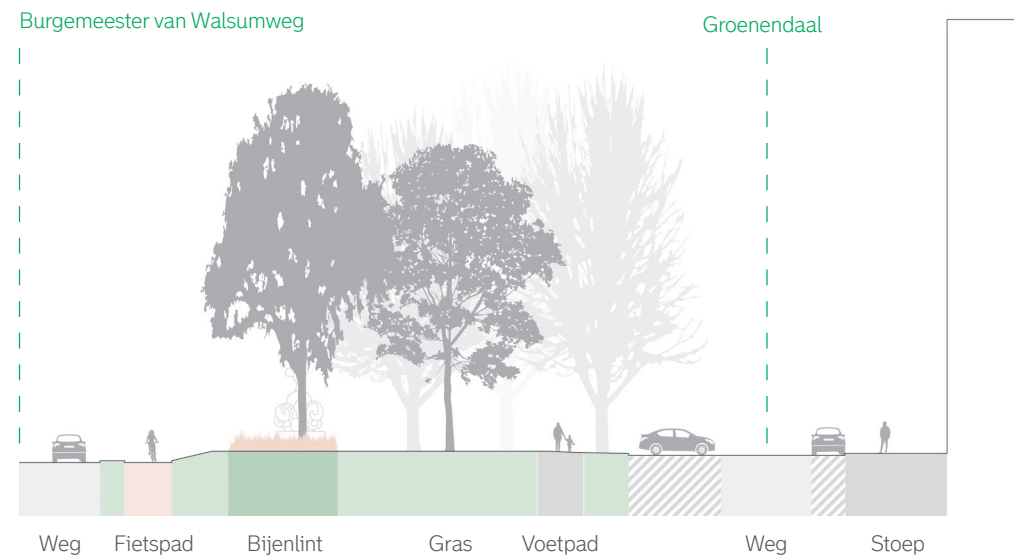
Een doorsnede vanaf de Burgemeester van Walsumweg tot aan de Groenendaal (Doorsnede 1b)
